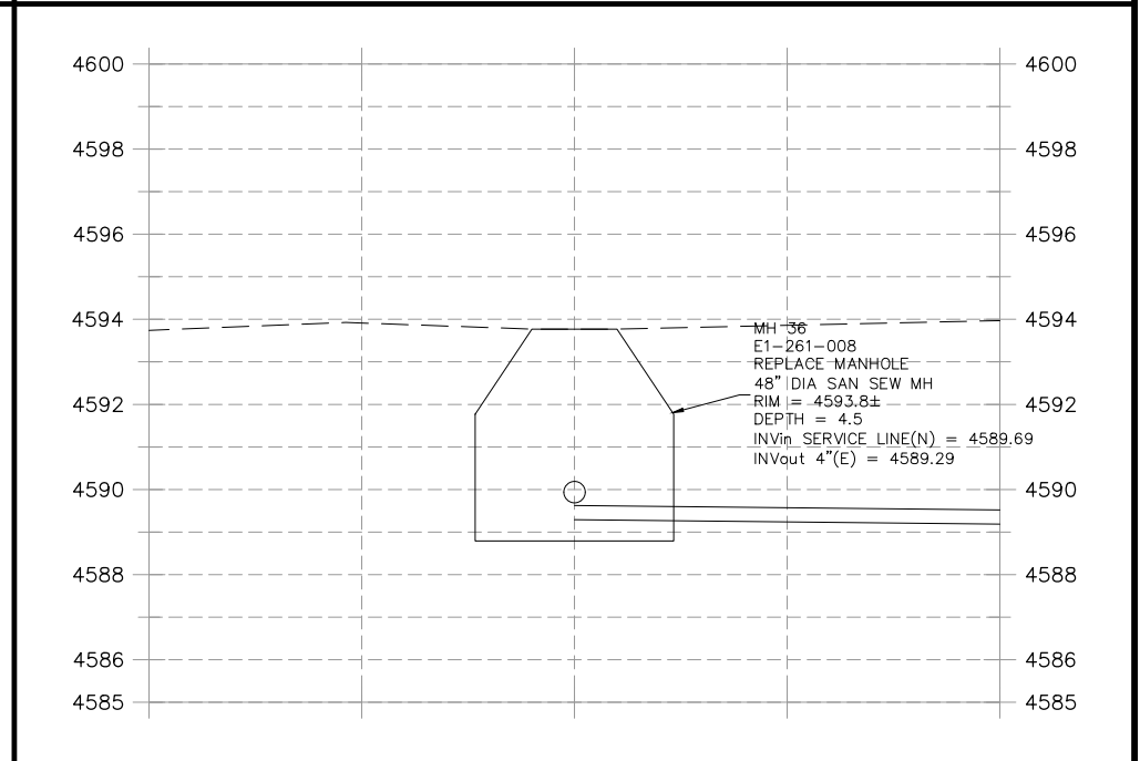
3 MANHOLE 36
