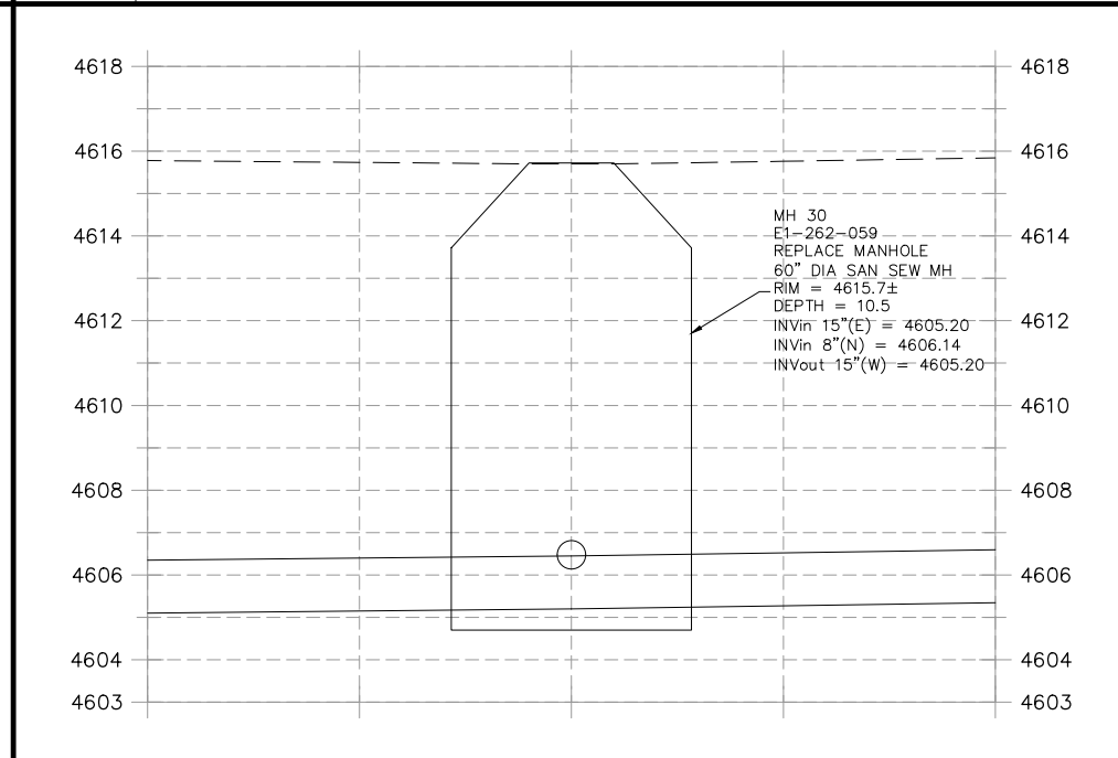
2 MANHOLE 30
