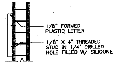
⑤ SIGNAGE SECTION N.T.S.
